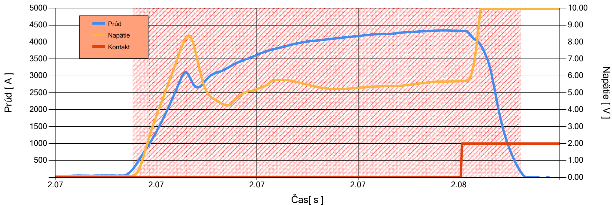
Dynamická skúška
